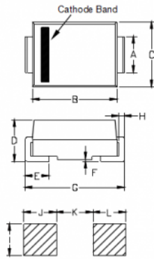
DO-214AC (SMA)
